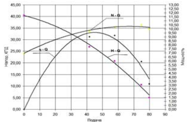
Рабочая характеристика ( \gamma=1000\text{кг/м}^3 , n=2900 об/мин)
