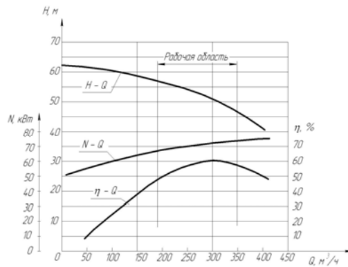
К 200-125-250Е с двигателем 75кВт
