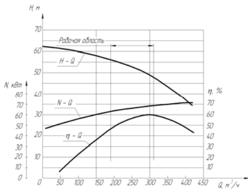
К 200-125-250Е - Б с двигателем 55кВт
