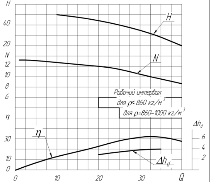
Характеристики АВС-80 испытанных на воде с плотностью \rho=1000 \text{ кг/м}^3 , при частоте вращения 1450об/мин
