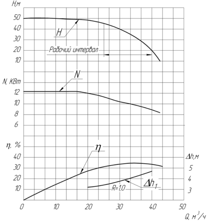
Характеристики 1АСВН-80А испытанных на воде с плотностью \rho=1000 \text{ кг/м}^3 , при частоте вращения 1450об/мин
